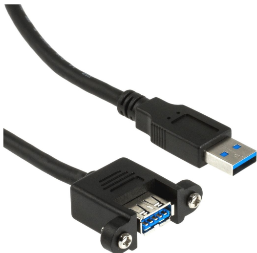
Schraubentyp UNC 4-40
