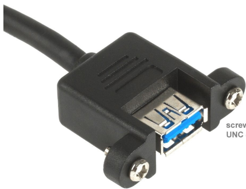
Schraubentyp UNC 4-40
